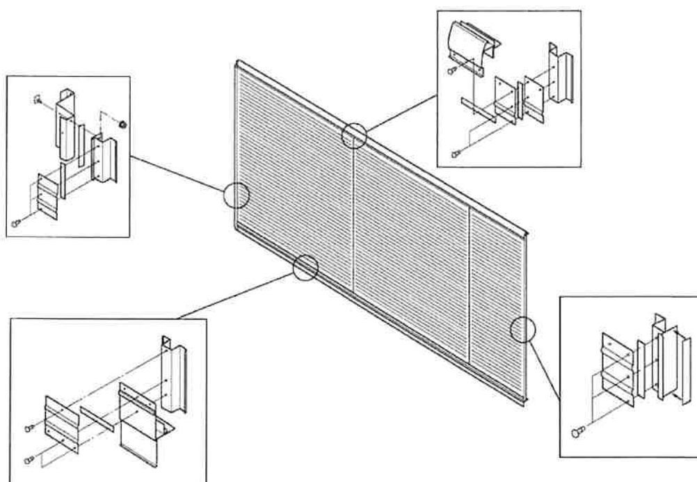
サイドパネル（フロントパネルも同様）
