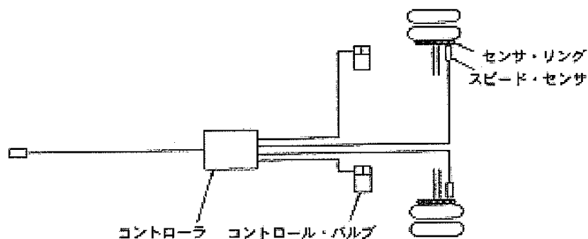
ABS用電氣配線図
