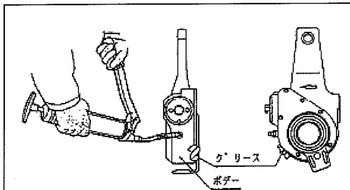
給脂要領
