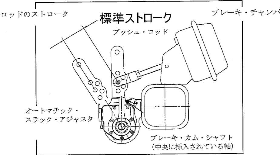
ブレーキ装置概要
